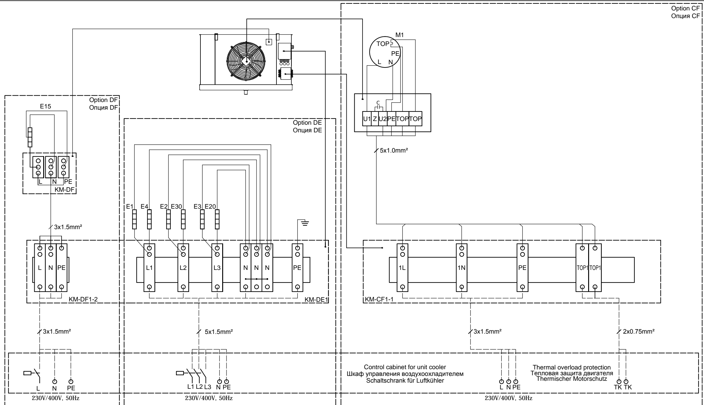
Drain line heater Нагреватель сливной магистрали Taufwasserheizung
